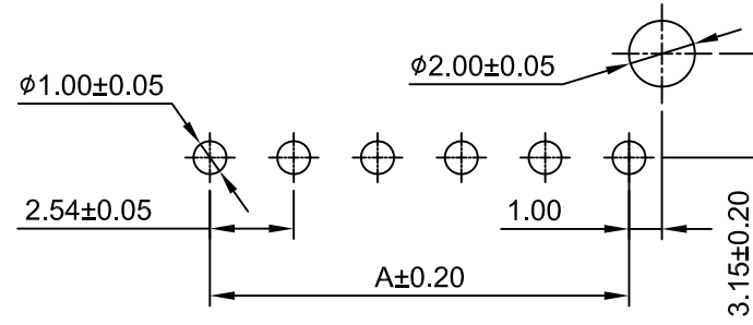
P.C.B LAYOUT
