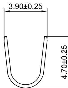
SEC:A-A
