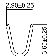
SEC:B-B
