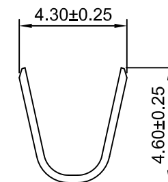
SEC:A-A
