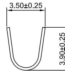
SEC:A-A
