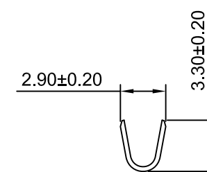
SEC:B-B
