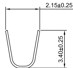
SEC:A-A
