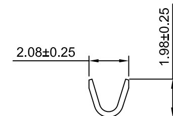
SEC:B-B
