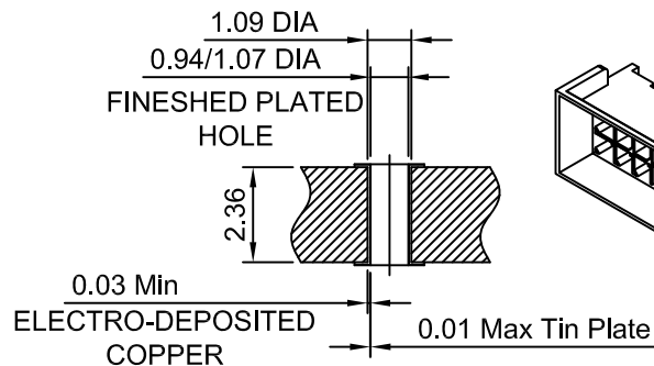
SEC:A-A SCALE 2.5:1
