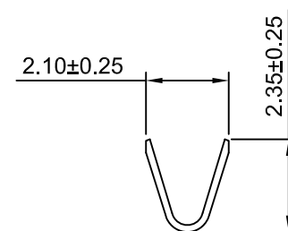
SEC:A-A
