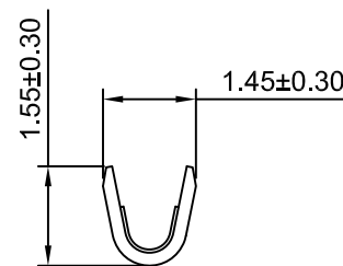
SEC:B-B
