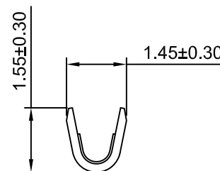
SEC:B-B
