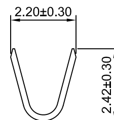
SEC:A-A
