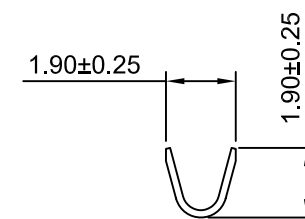
SEC:A-A
