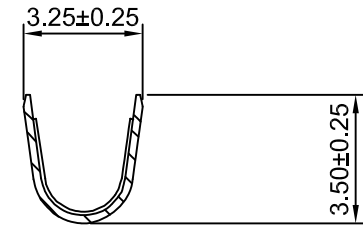
SEC:A-A
