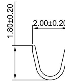
SEC:A-A
