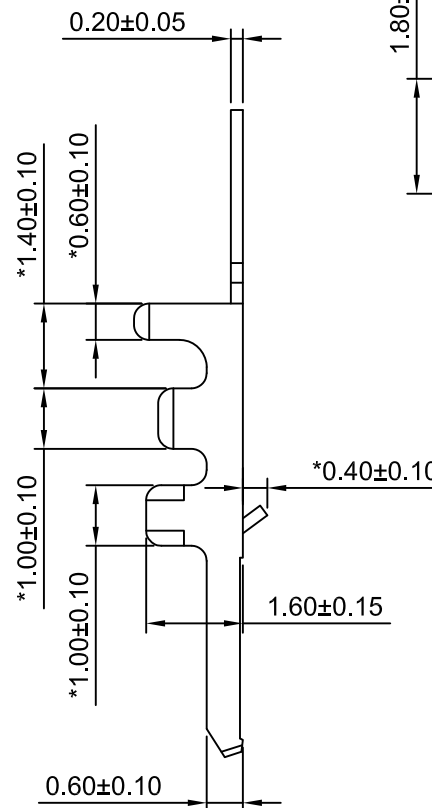
SEC:A-A
