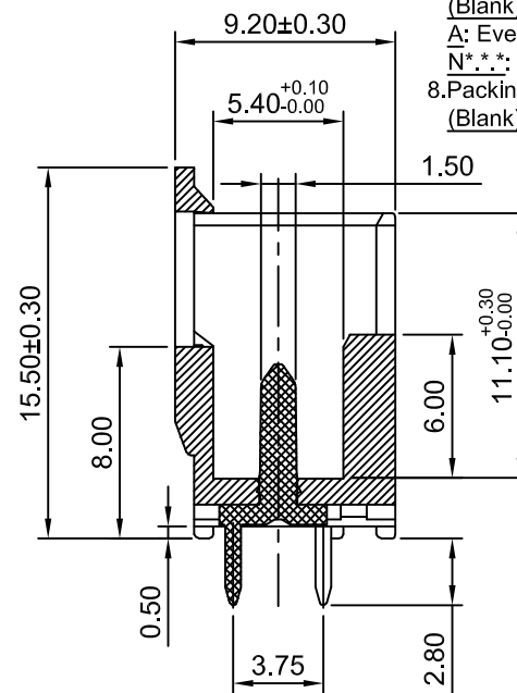
SEC: A-A
