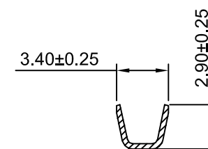
SEC:B-B
