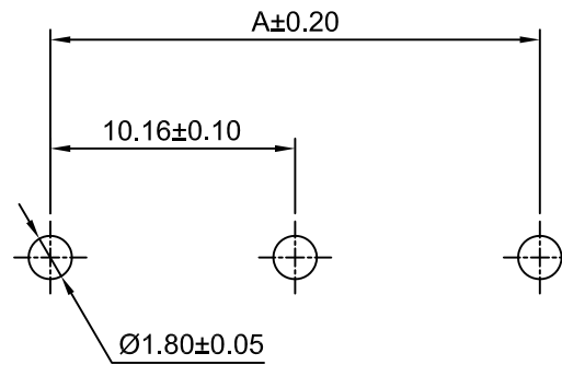
P.C.B LAYOUT
