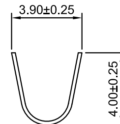
SEC:A-A
