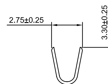
SEC:B-B
