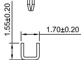
SEC:A-A
