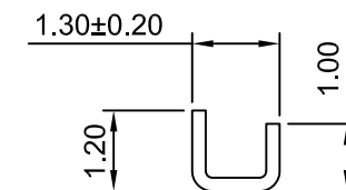
SEC:A-A
