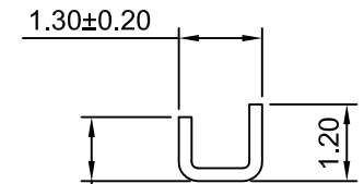
SEC:B-B
