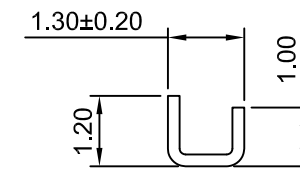
SEC:A-A
