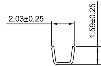
SEC:A-A
