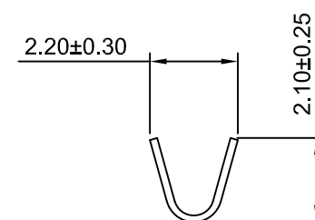
SEC:A-A
