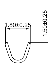
SEC:B-B
