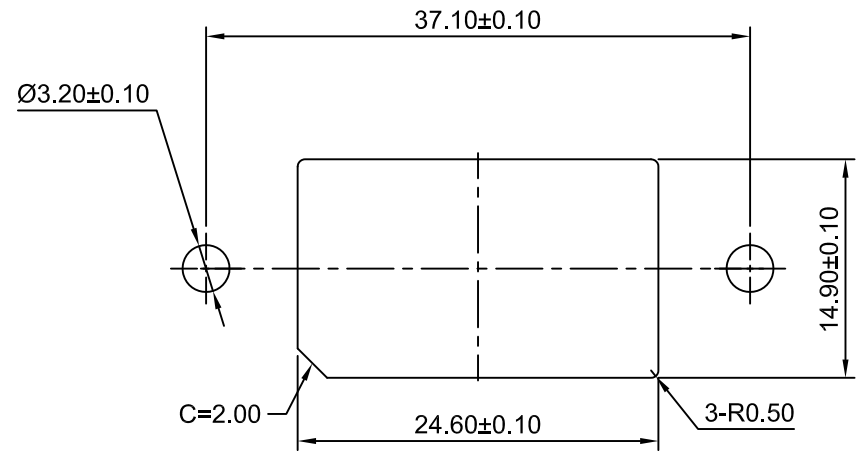
P.C.B LAYOUT
