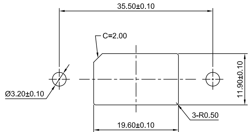
P.C.B LAYOUT
