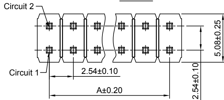
SEC:A-A
