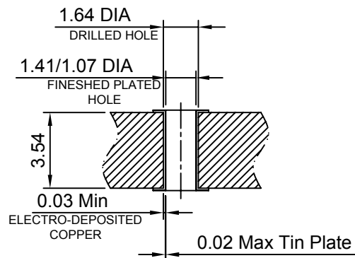
SEC:A-A
