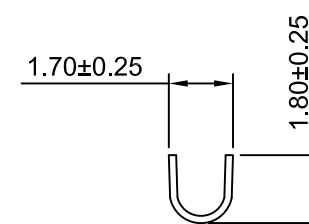
SEC:B-B
