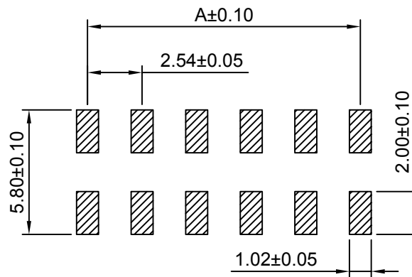
P.B.C LAYOUT
