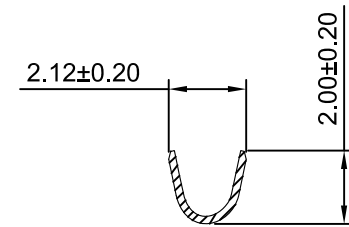
SEC:A-A
