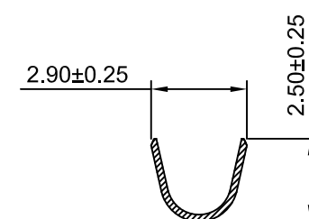
SEC:A-A
