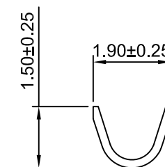
SEC:B-B
