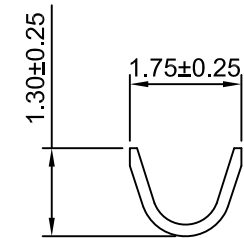
SEC:B-B
