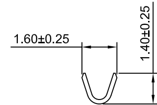
SEC:B-B
