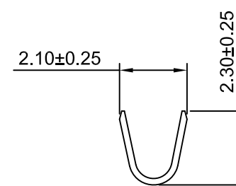
SEC:A-A
