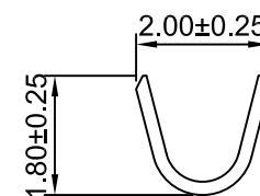
SEC:B-B
