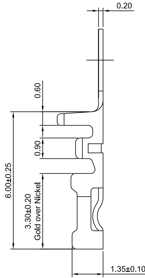
SEC:A-A
