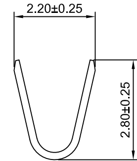
SEC:A-A
