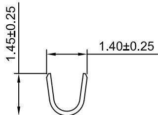
SEC:B-B
