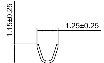
SCE: B-B
