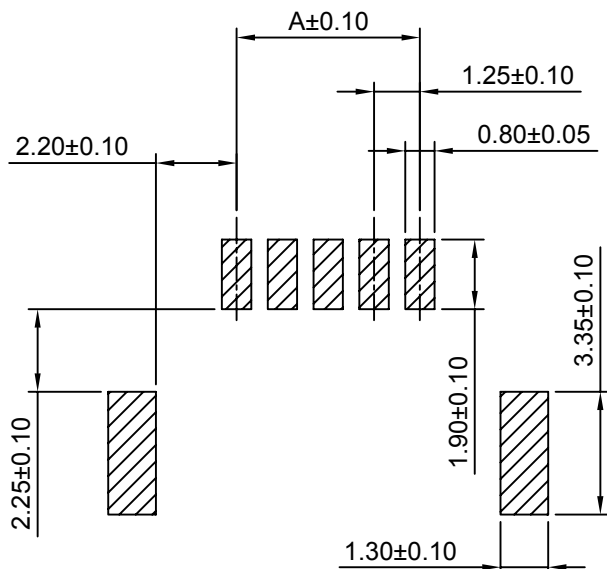
P.C.B. LAYOUT
