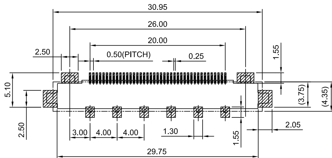
P.C.B LAYOUT
