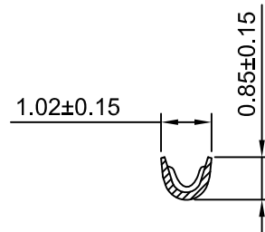
SEC:B-B
