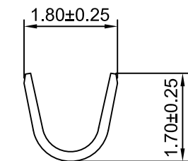
SEC:B-B
